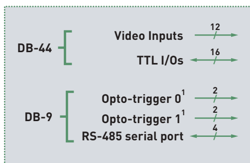
I/O module
